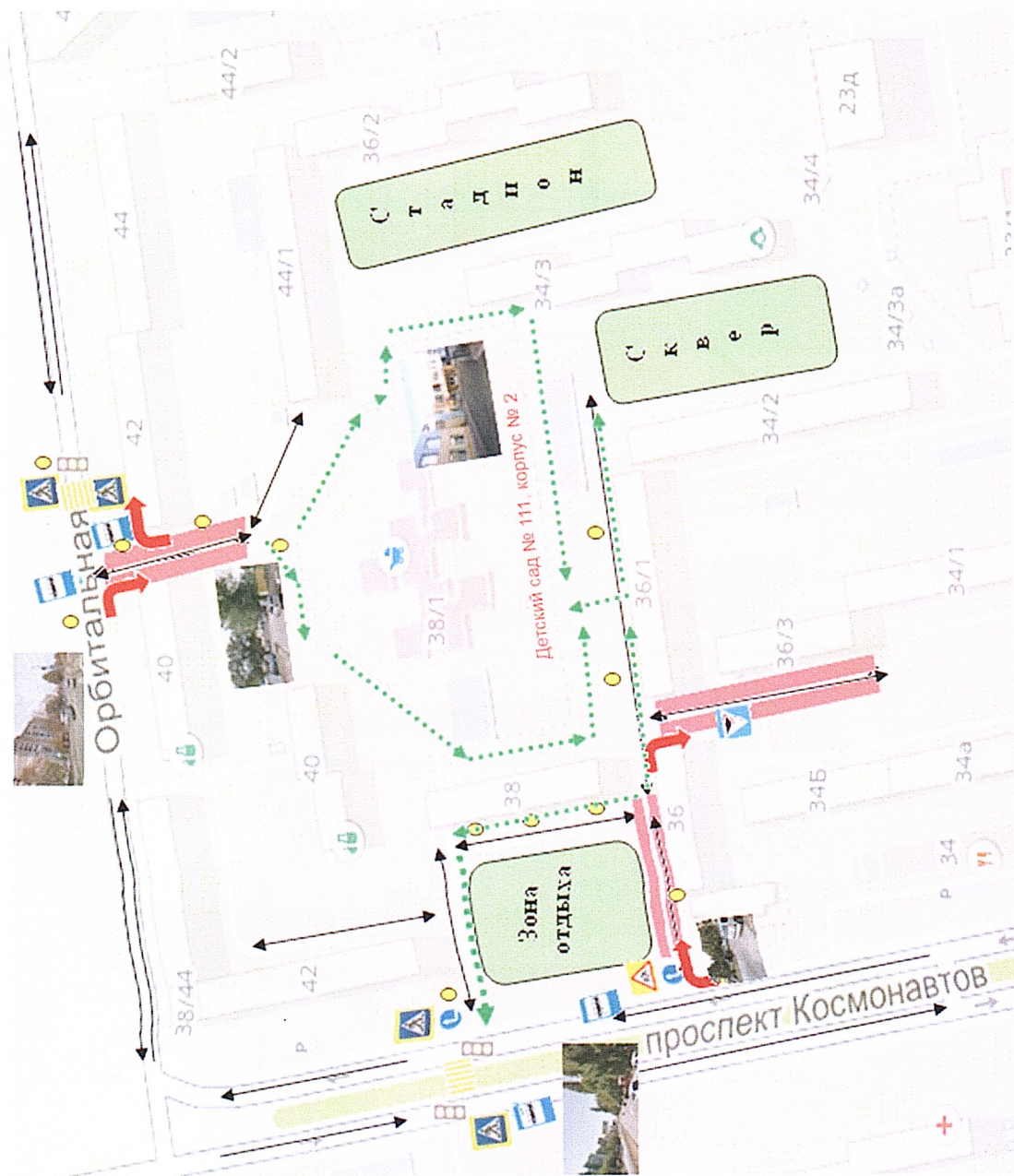
2. Схема организации дорожного движения в непосредственной близости от образовательной организации с размещением соответствующих технических средств организации дорожного движения, маршрутов движения детей и расположения парковочных мест
